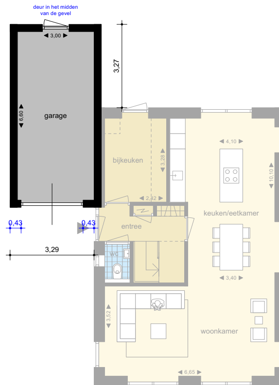
Type 1 - inwendig 3,00 x 6,60 m
