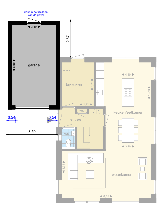
Type 3 - inwendig 3,30 x 6,00 m
