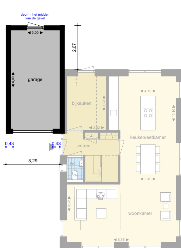
Type 1 - inwendig 3,00 x 6,00 m
