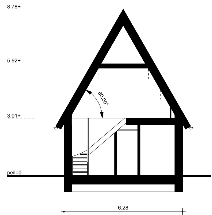
doorsnede
