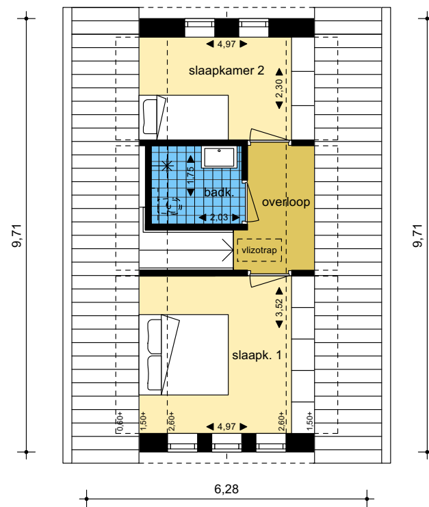
1e verdieping
