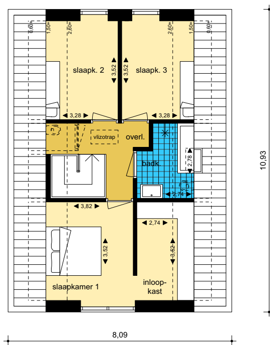
1e verdieping
