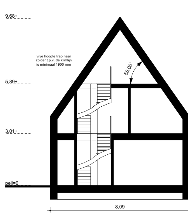
doorsnede
