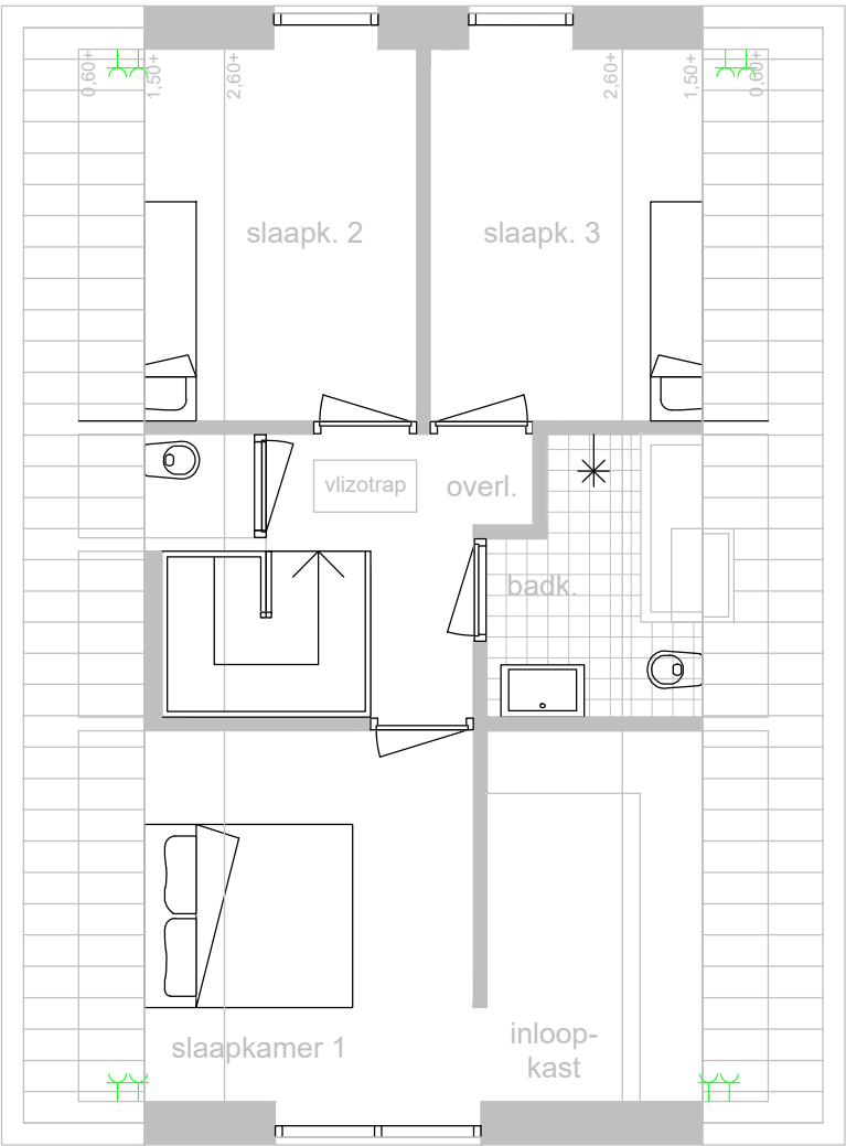
1e verdieping
