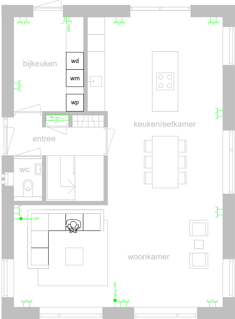
begane grond
