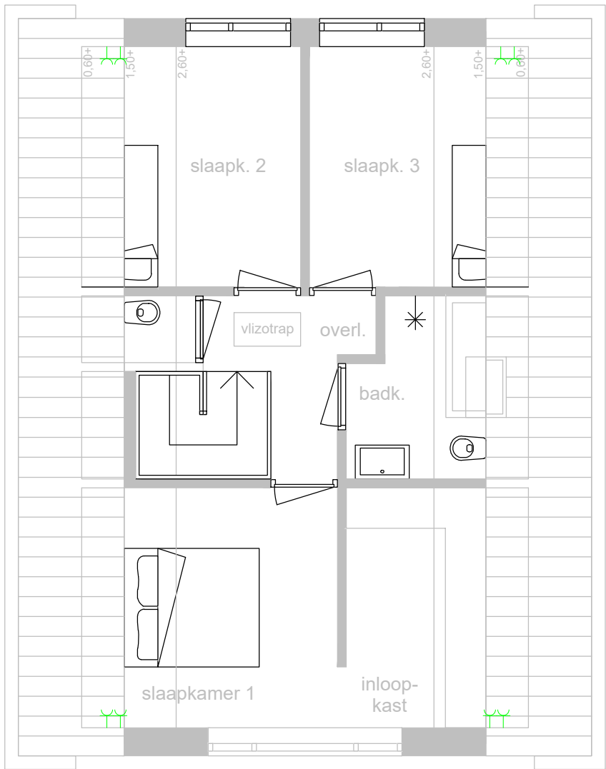
1e verdieping
