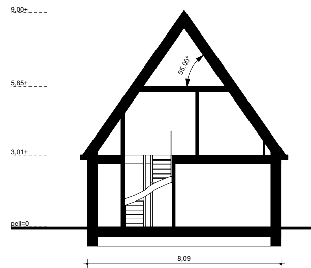
doorsnede
