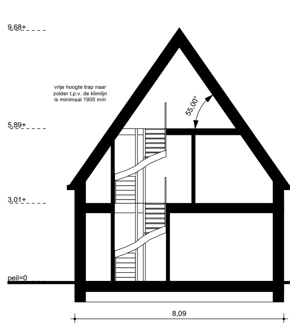
doorsnede
